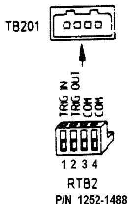
図3-10. トリガ・コネクタ
