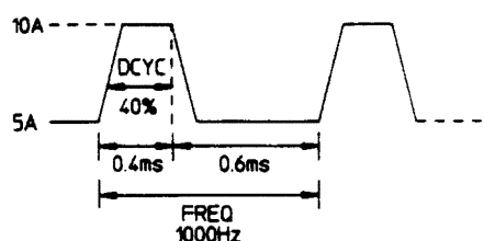
図2-4. 連続トランジェント操作
