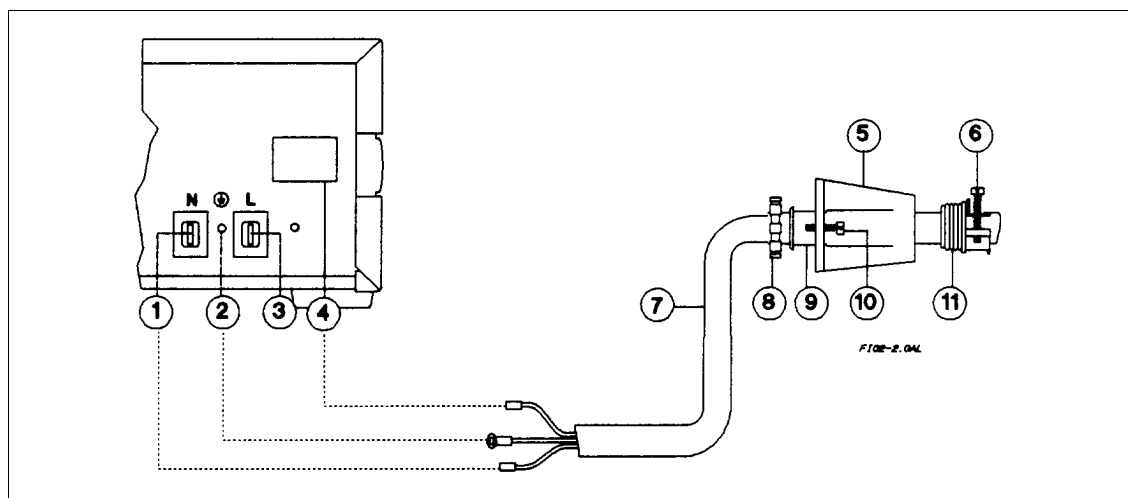
図2-2. シリーズ667xA電源コードの接続
