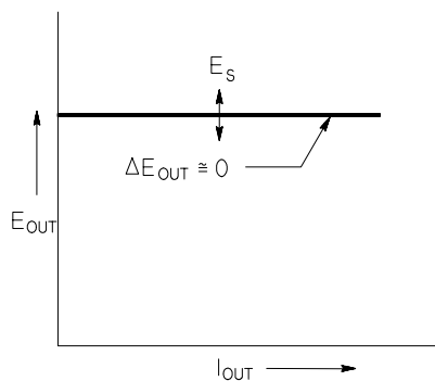
图 7-3. 理想的恒压电源
