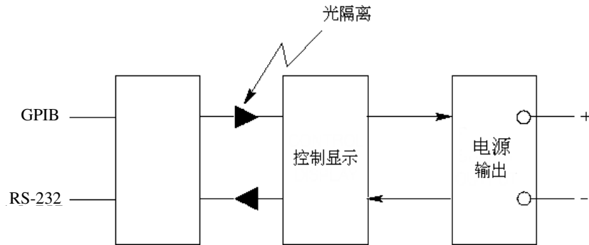
图 7-2. 示意光隔离的电源简图
