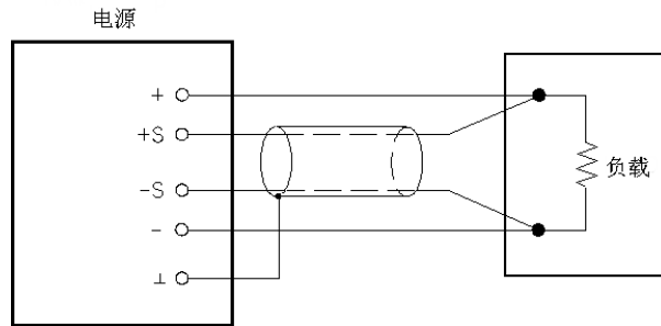
图 3-2. 远程电压检测连接
