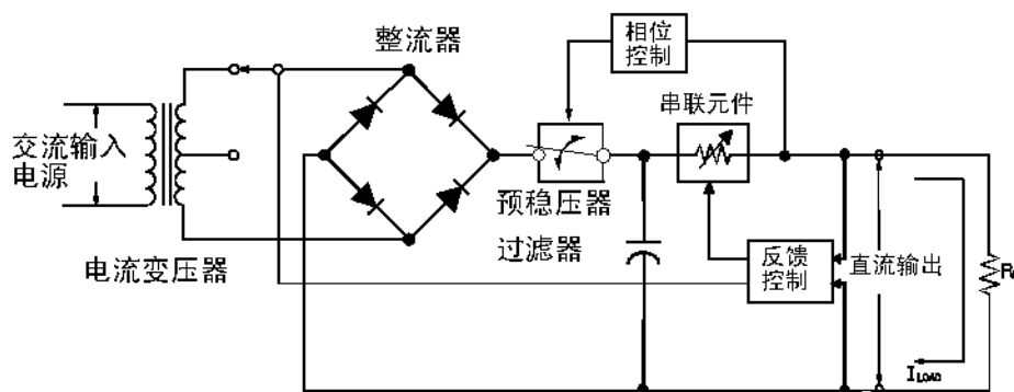
图 7-1. 简单的串连电源示意图
