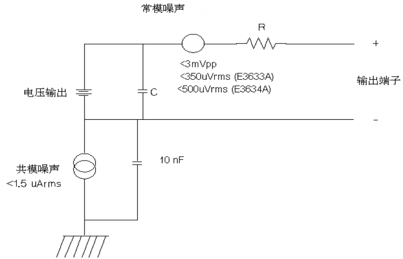
图 7-6. 共模和常模噪声源简图
