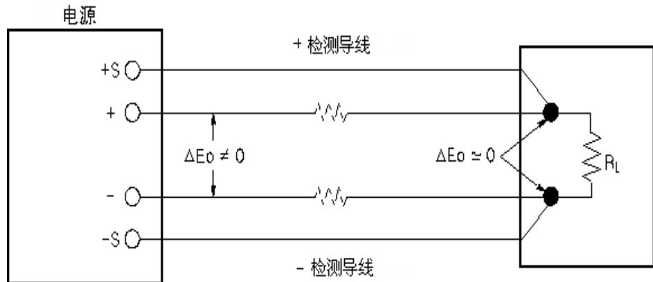
图 7-7. 进行远程检测的稳压电源
