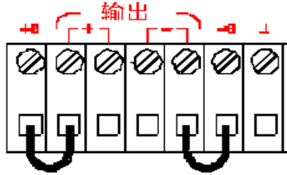
图 3-3. 后面板本地检测连接
