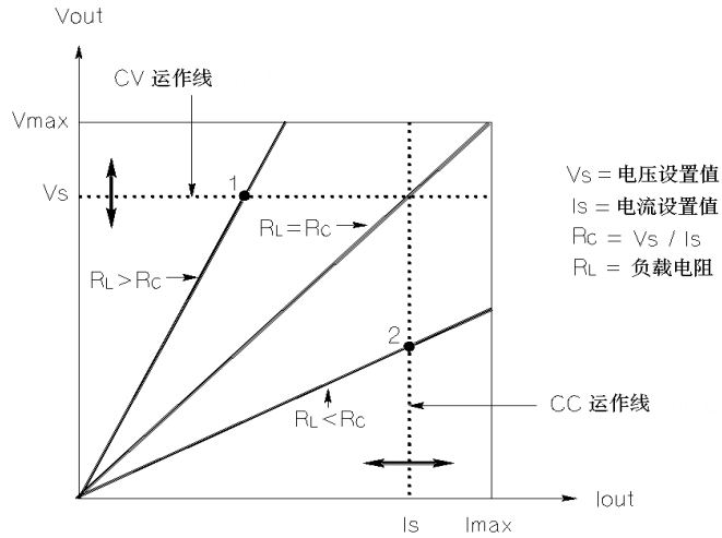
图 7-5. 输出特性
