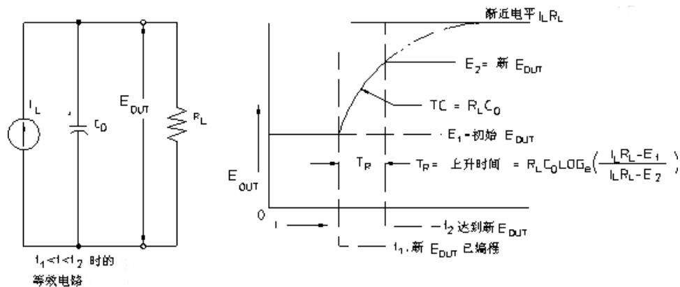
图 7-8. 响应速度——电压上升的编程（满载）
