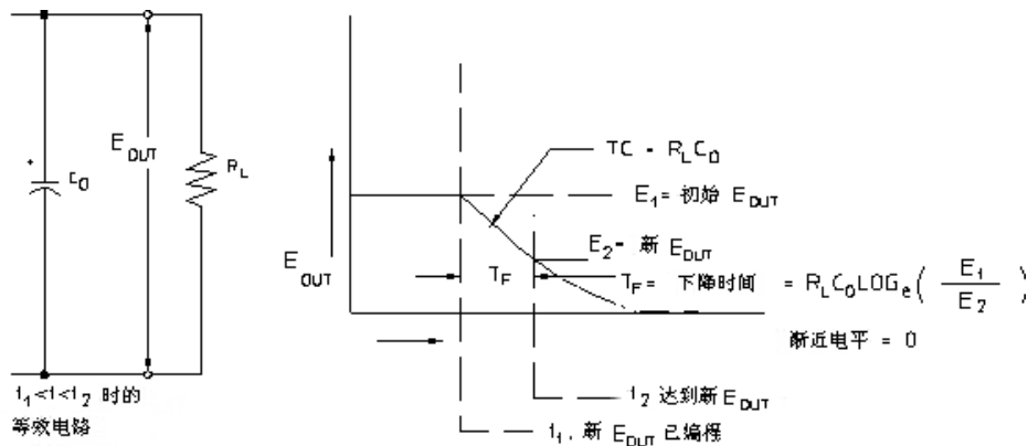
图 7-9 响应速度——电压下降的编程
