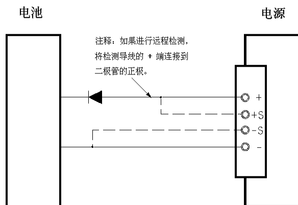
图 3-1. 建议的电池充电保护电路
