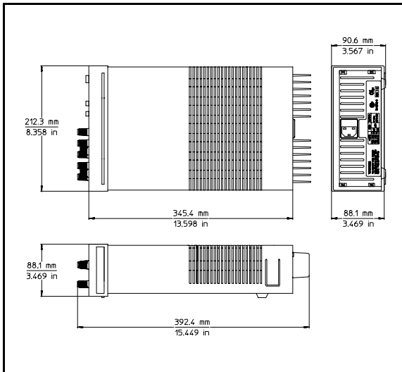
그림 1. 외형도
